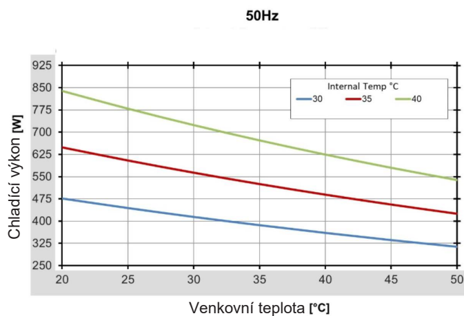
Chladicí výkon v závislosti na teplotě
