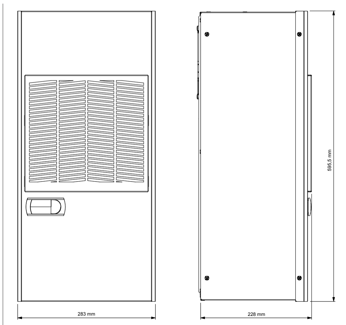
Technický výkres
