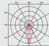
FUTURA NB 2.4ft (s mřížkou)
