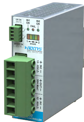
Redundancy Module
