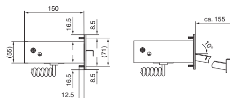
Montážní výřez
