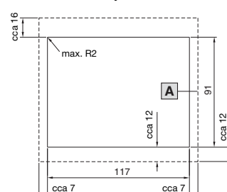
Montážní výřez
