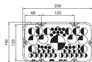
Velikost 1
