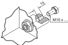
Upevnění z vnější strany
