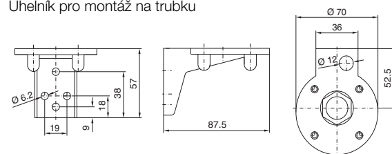
Úhelník pro montáž na trubku
