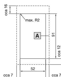
Montážní výřez
