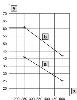
Graf odolnosti proti zkratu 9340.000/9340.050
