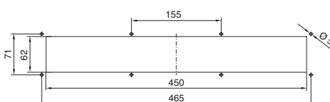
Montážní výřez
