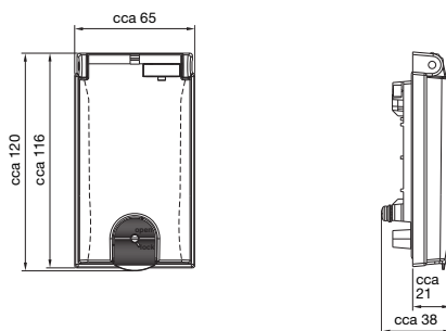
Sklopný kryt rozhraní dvojité
