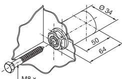
Upevnění z vnitřní strany
