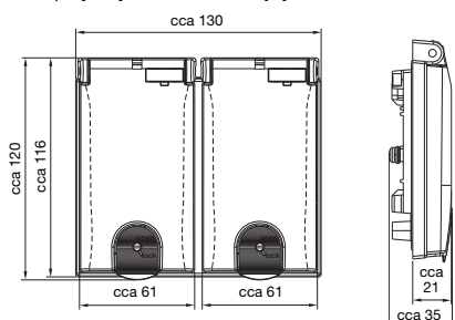
Sklopný kryt rozhraní dvojité
